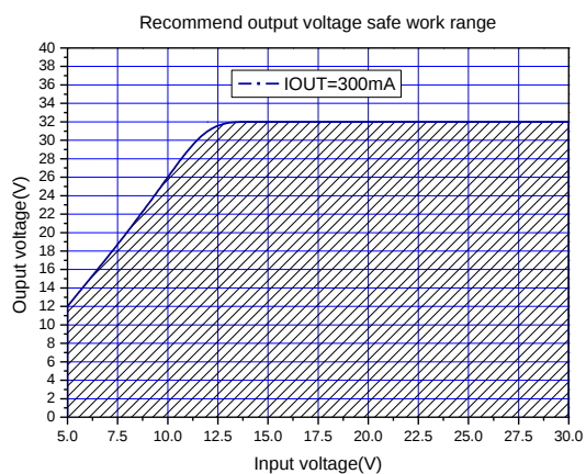
图 7.最大输出电压(IOUT=300mA)
