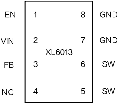
图 2. XL6013 引脚配置
