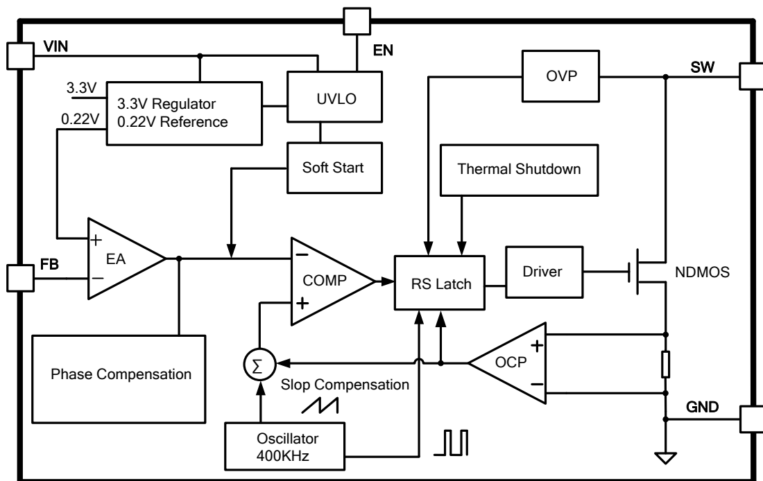
图 3. XL6013 方框图
